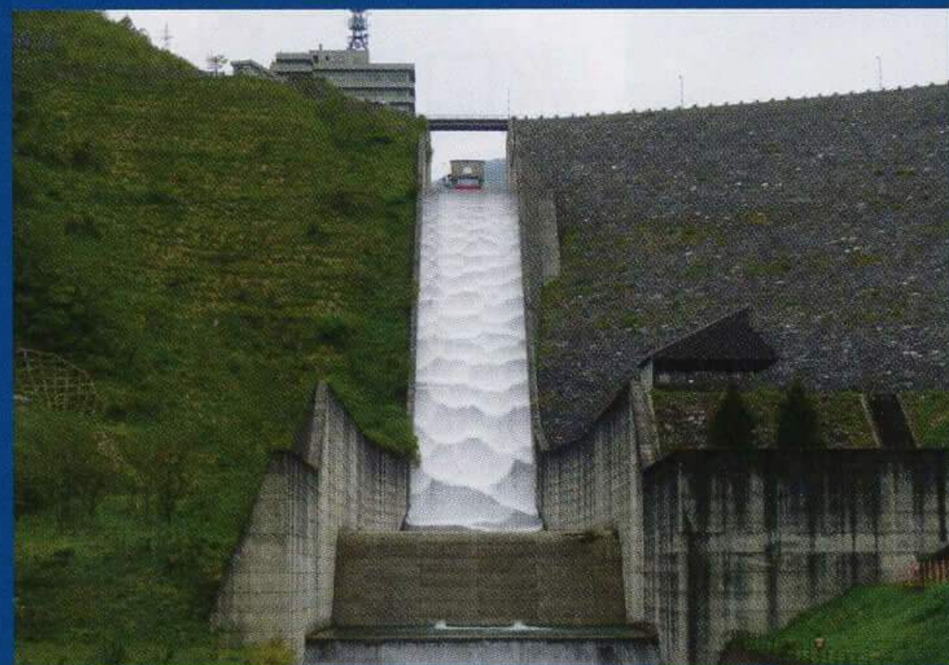
土や石を積み上げたロックフィルダムという型式の三国川ダム
