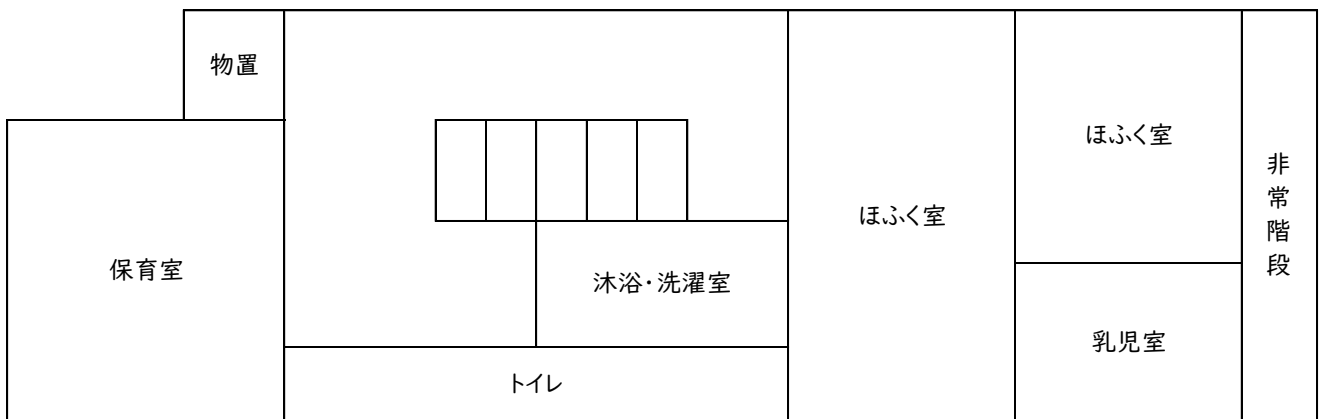
1階平面図
